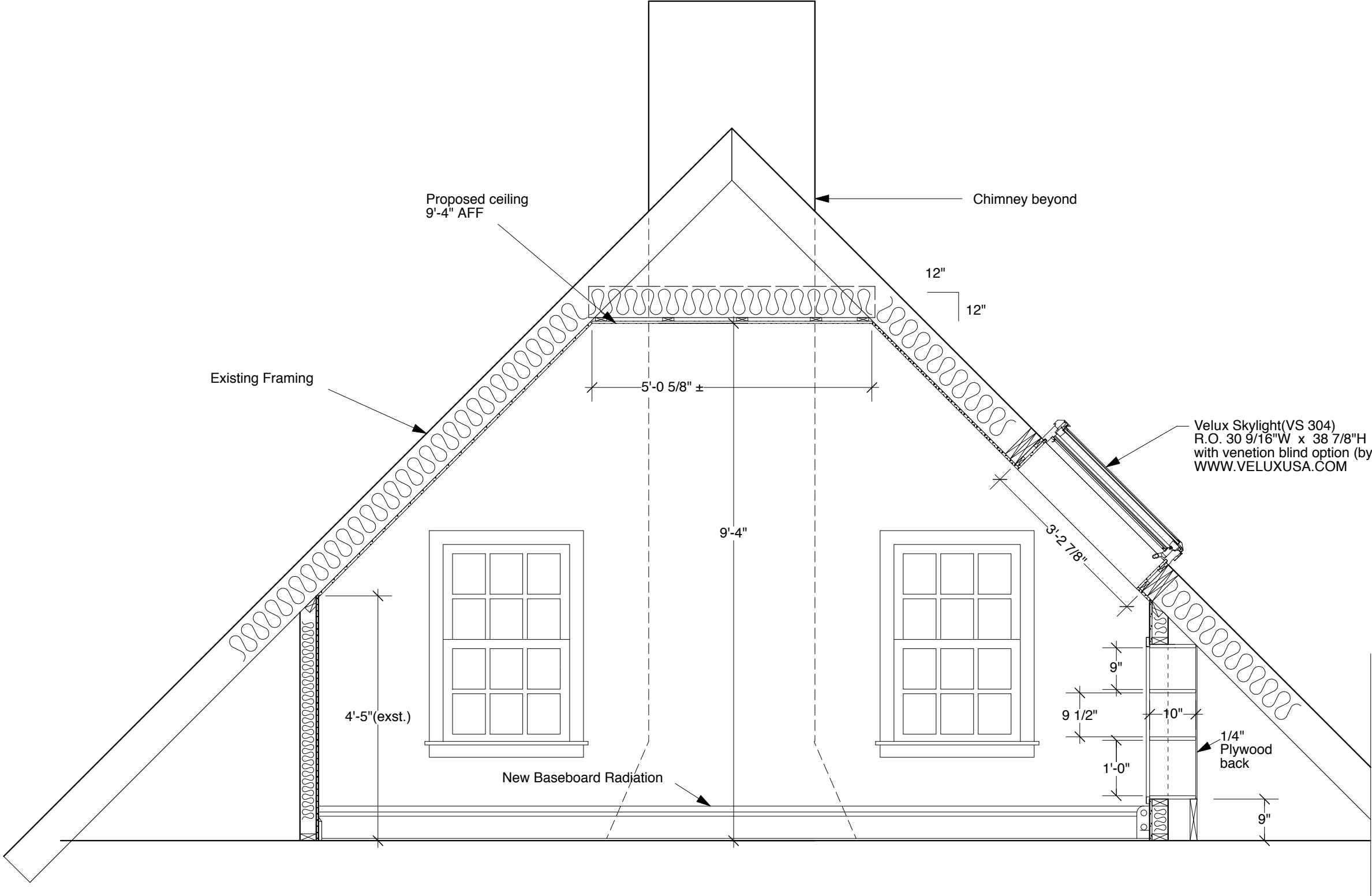
2 Section A-A Scale: 1/2" = 1'-0"
